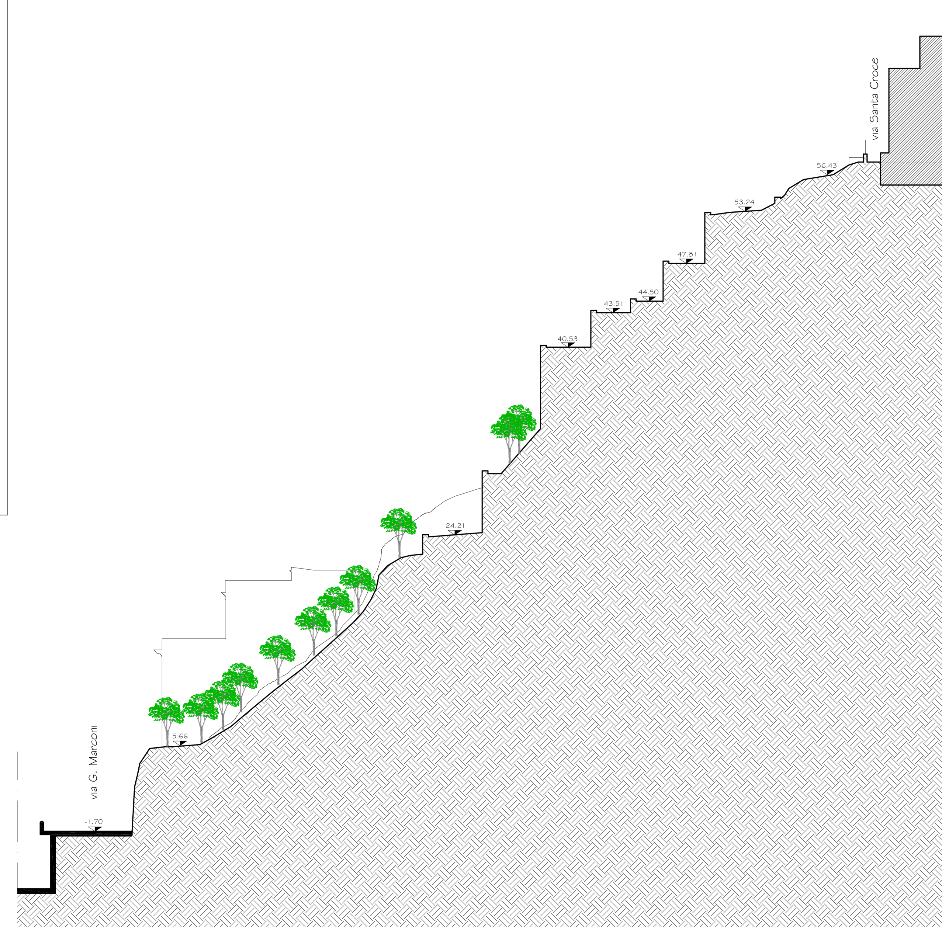
PROFILO - STATO ATTUALE SCALA 1:200
