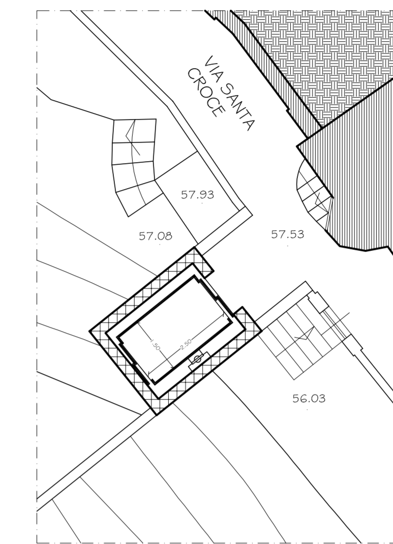
PIANTA - PROGETTO SCALA 1:100
