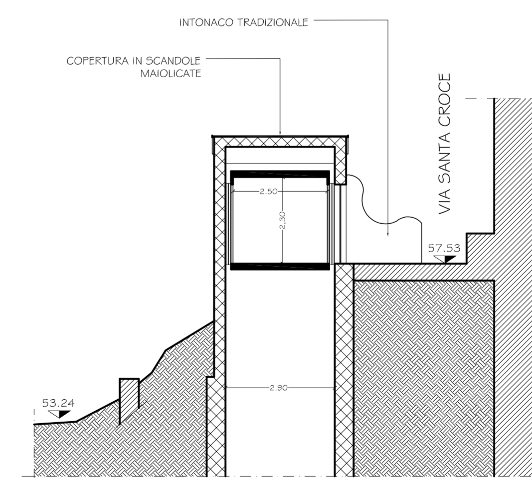
SEZIONE - PROGETTO SCALA 1:100
