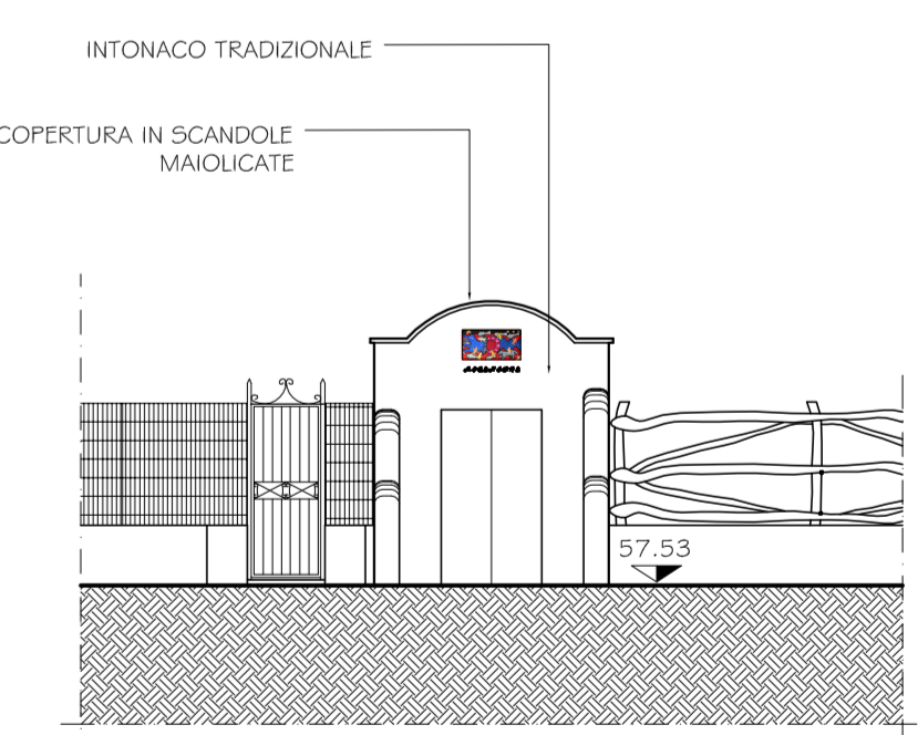
PROSPETTO - PROGETTO SCALA 1:100
