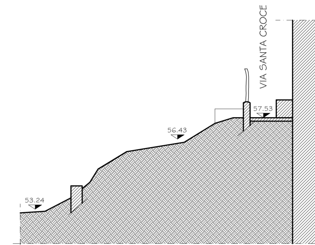
SEZIONE - STATO ATTUALE SCALA 1:100
