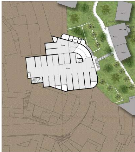
PLANIMETRIA PIANO QUARTO INTERRATO D=242,90
